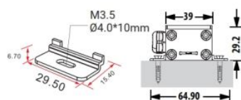
Montagehalter
