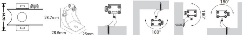
Schwenkbarer Halter
