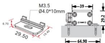
Montagehalter
